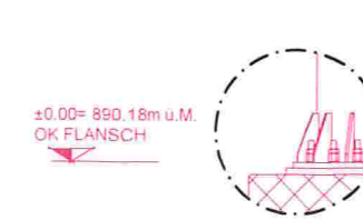
DETAIL NULLPUNKT (1:50)
