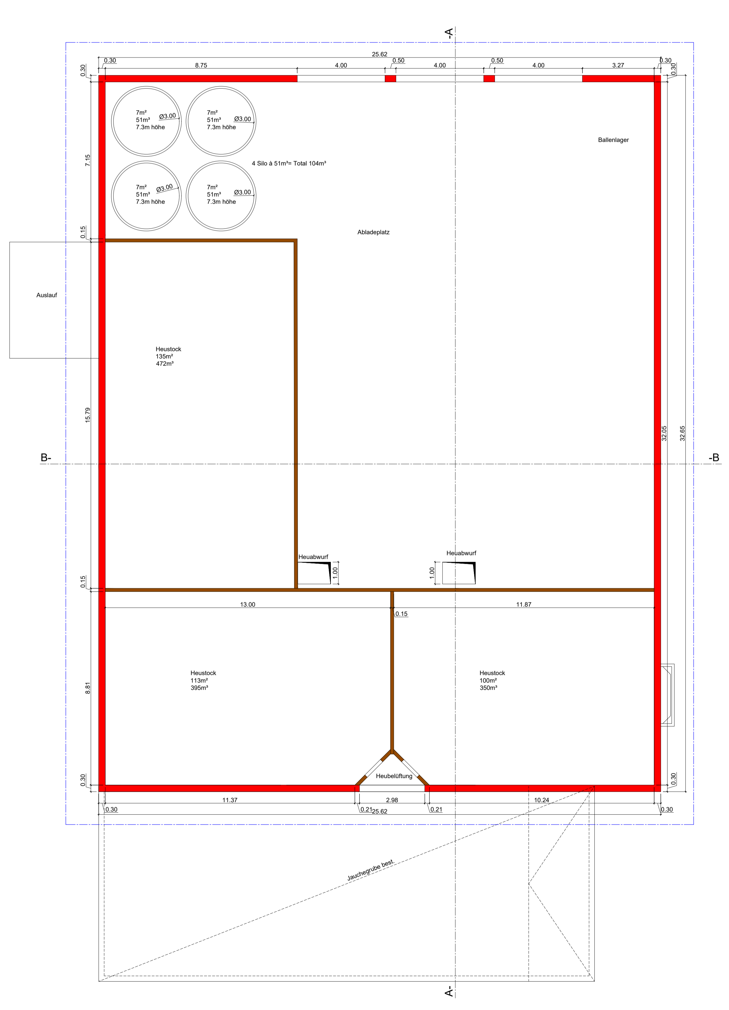
Grundriss OG
