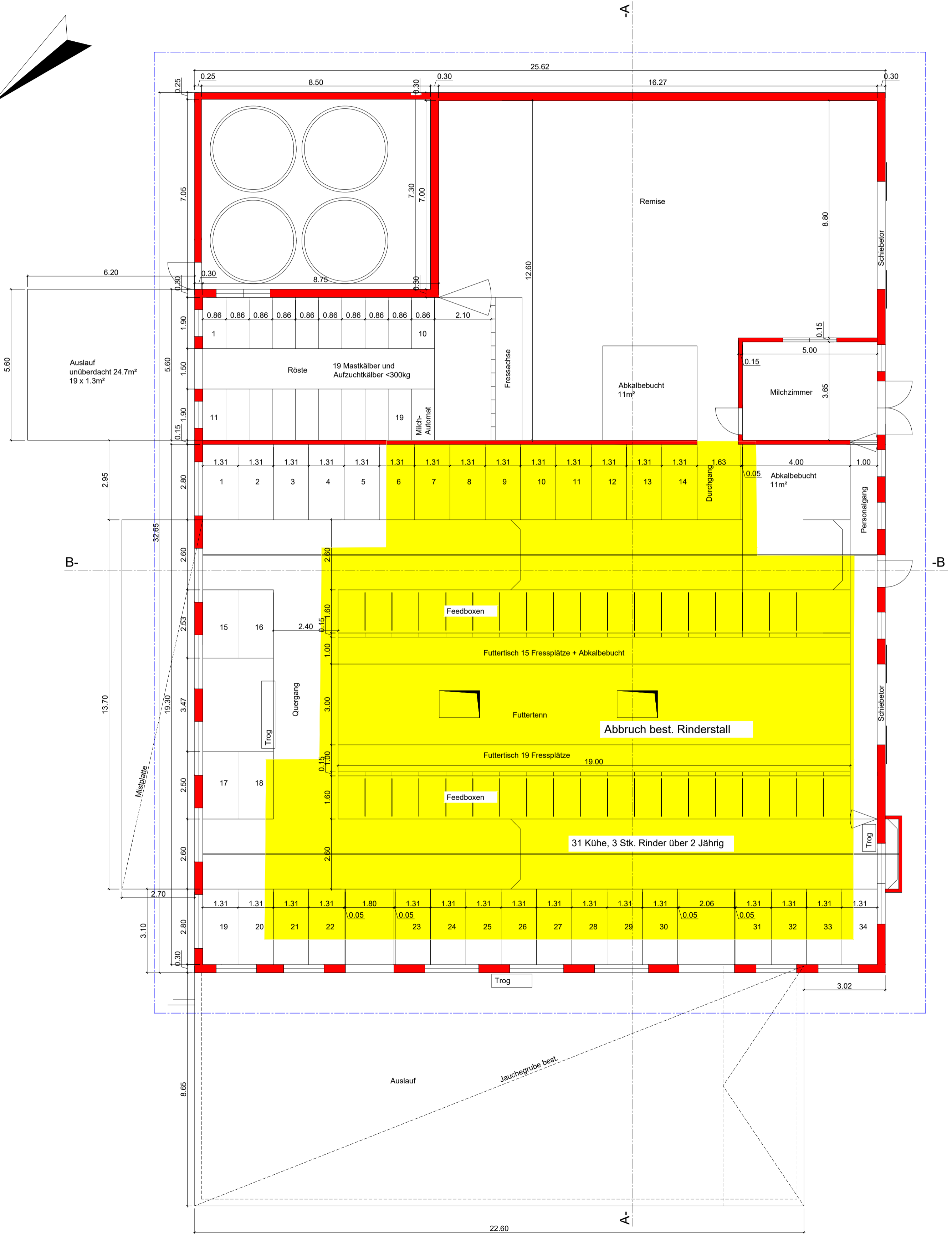
Grundriss EG
