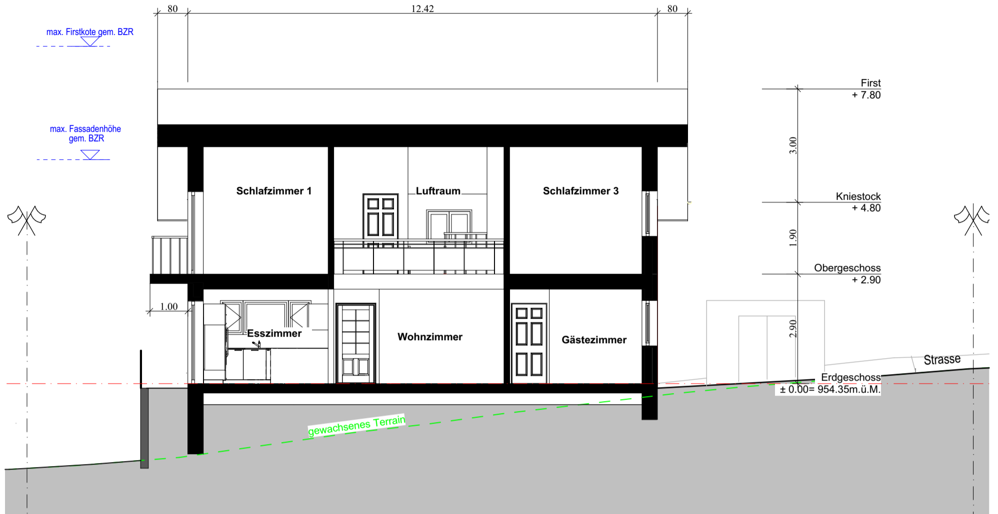
Längsschnitt
