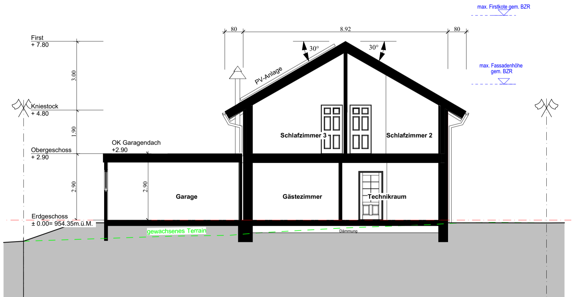
Querschnitt
